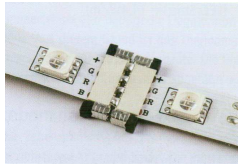
LED36-CON Verbiner
